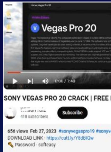
INFOSTEALER
