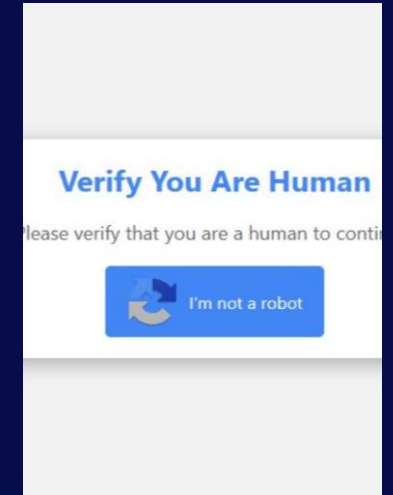
CLICKFIX
